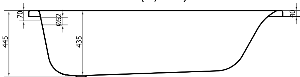
A-A ( 0,1 : 1 )
