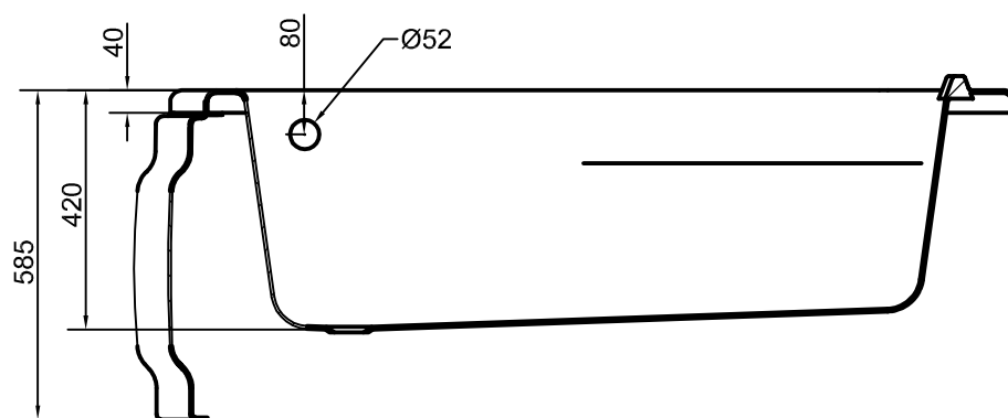
A-A ( 1 : 10 )
